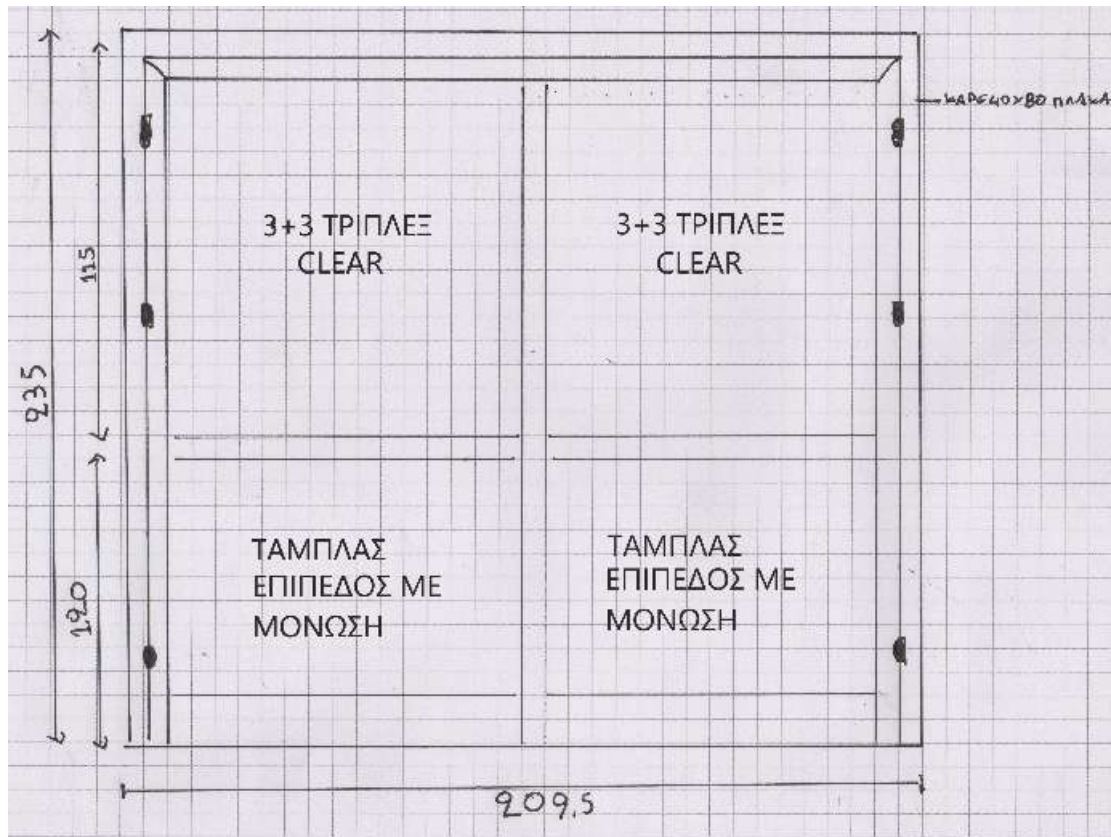
ΕΝΔΕΙΚΤΙΚΟ ΣΚΑΡΙΦΗΜΑ
